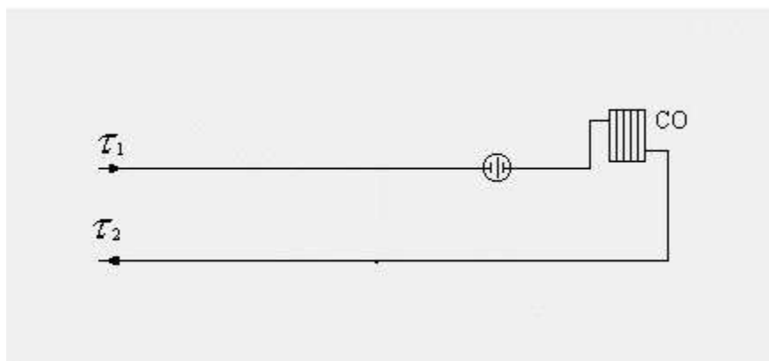
Рисунок 1.3.1. Схема присоединения теплотребляющих установок потребителей к тепловым сетям
