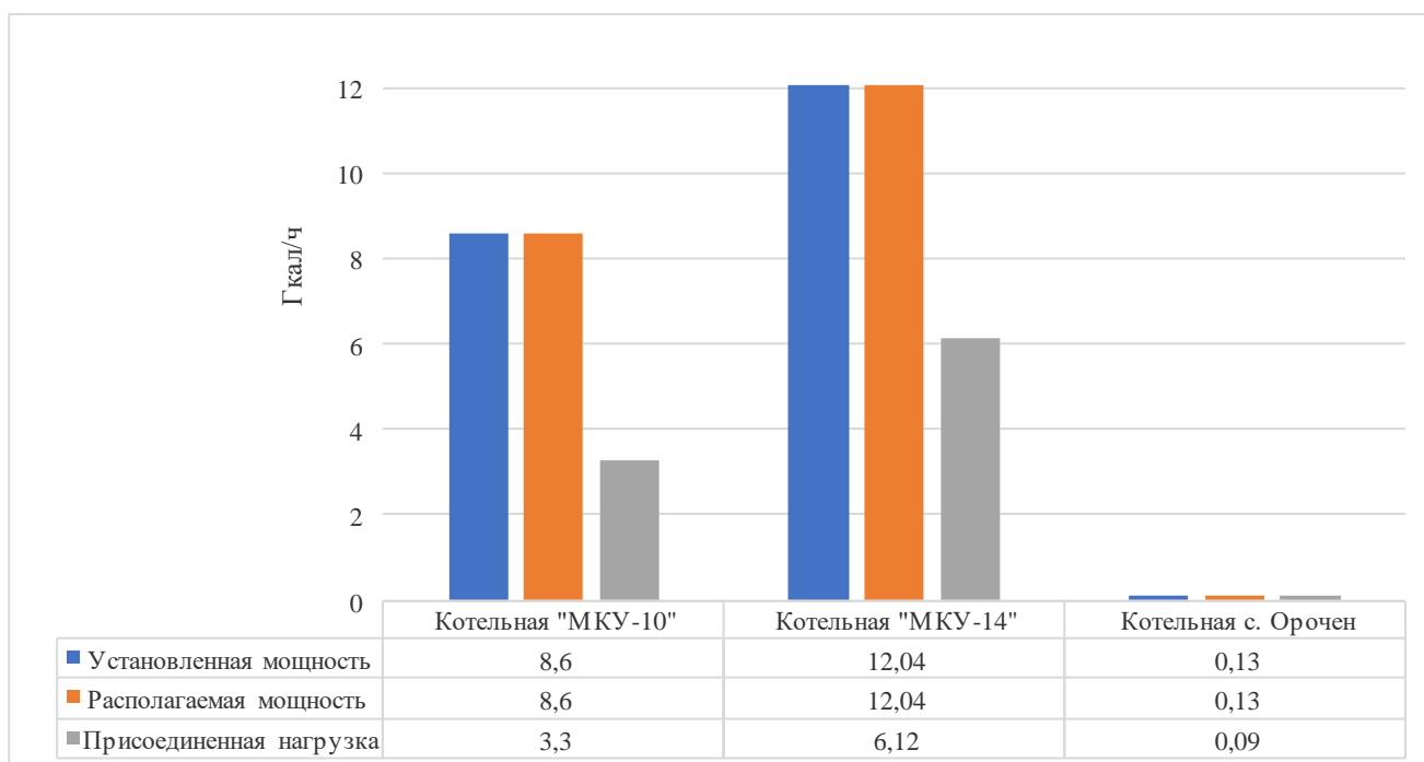
Рисунок 1.2.1 – Распределение мощностей источника тепловой энергии
