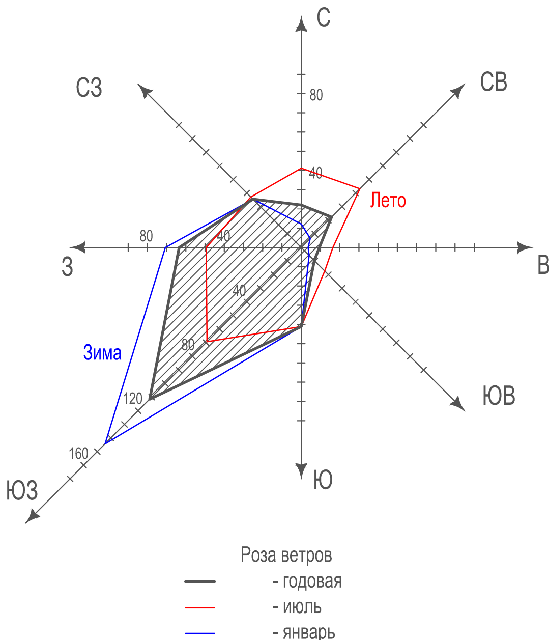
Роза ветров
